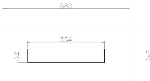
Måttskiss på monteringsplåt art.nr: 460418
